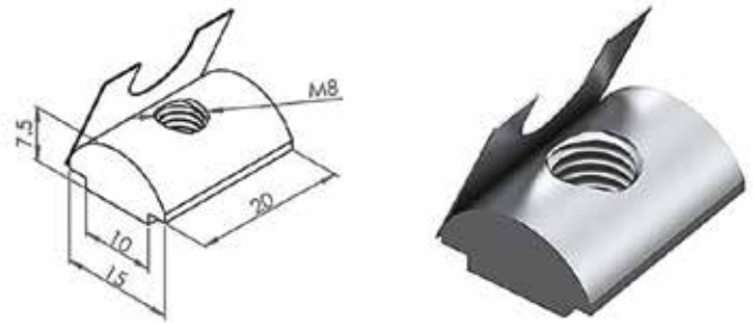
Modül T Somunu
